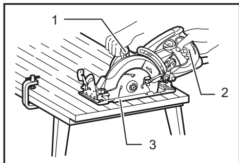
► 1. Agarradera frontal 2. Empuñadura trasera 3. Base
