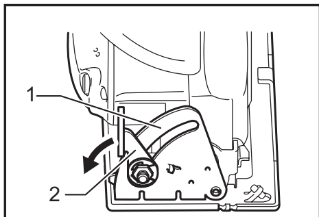
► 1. Plaque graduée de coupe en biseau 2. Levier
